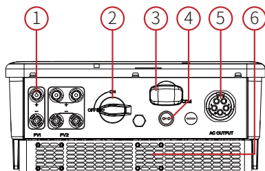
GW12KT-DT、GW15KT-DT
