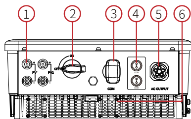
GW8K-DT、GW10KT-DT
